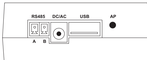
Rys.1 Układ gniazd przyłączeniowych w Module Internetowym
