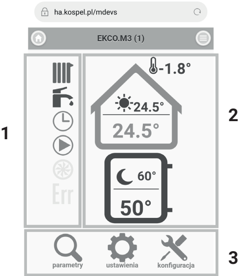
Rys.17 Ekran sterujący kotła z zasobnikiem
