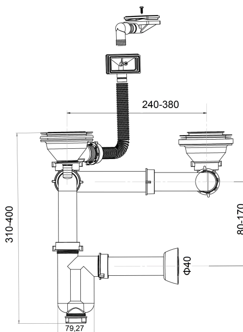
rysunek techniczny
