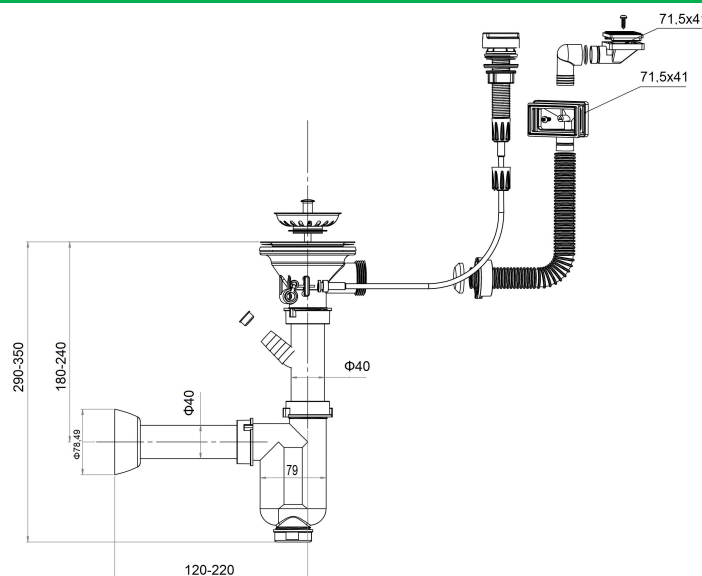
rysunek techniczny
