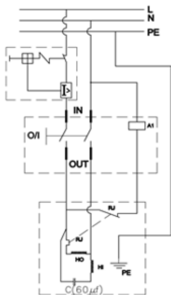
schemat obwodu elektrycznego
