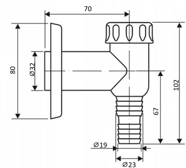
rysunek techniczny
