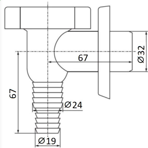
rysunek techniczny
