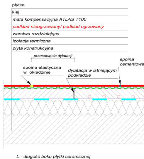
Rys. 1 Rozwiązanie tradycyjne - płytki ceramiczne ułożone na podkładzie z ogrzewaniem podłogowym i bez ogrzewania. Dylatacja w podłożu przeniesiona na posadzkę z płytek ceramicznych.
