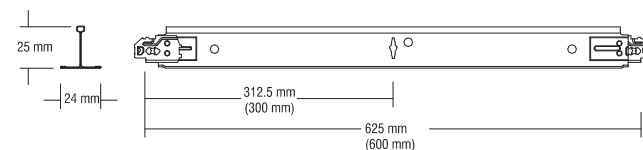
Profil poprzeczny krótki
