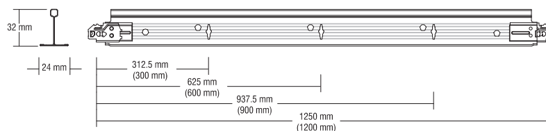
Profil poprzeczny długi
