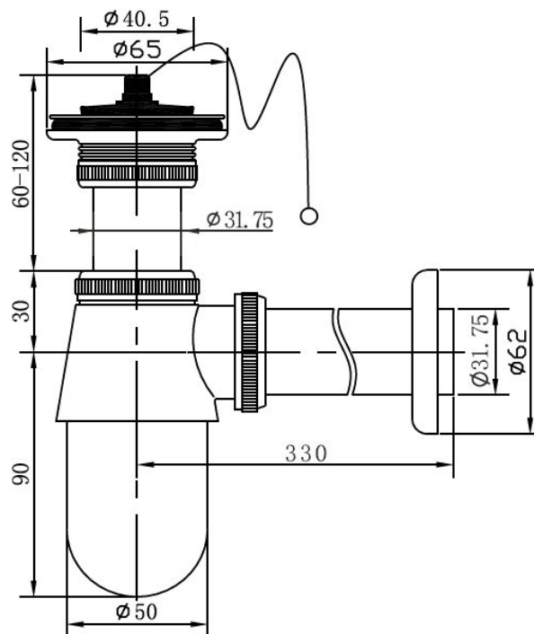
rysunek techniczny
