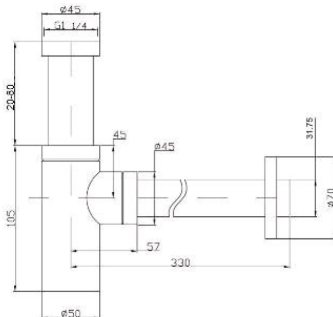
rysunek techniczny
